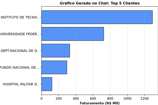
Figura 2: Agente Q&A com raciocínio ReAct, resposta em tabela estruturada e gráfico gerado dinamicamente.
